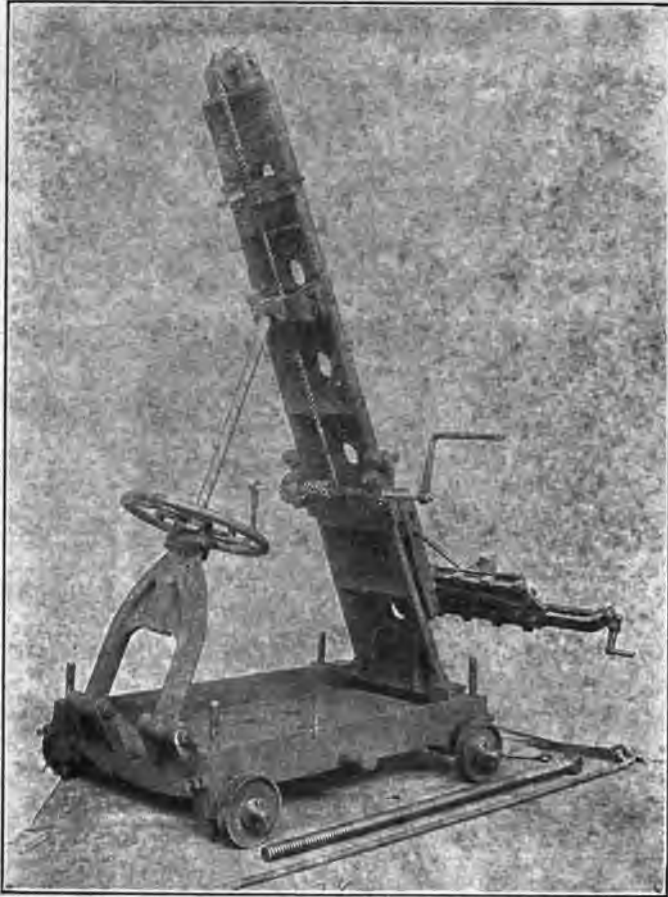
Fig. 26. Ingersoll-Sergeant Gadder.
